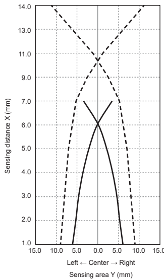
● PRD(L)18-7D□/14D□
